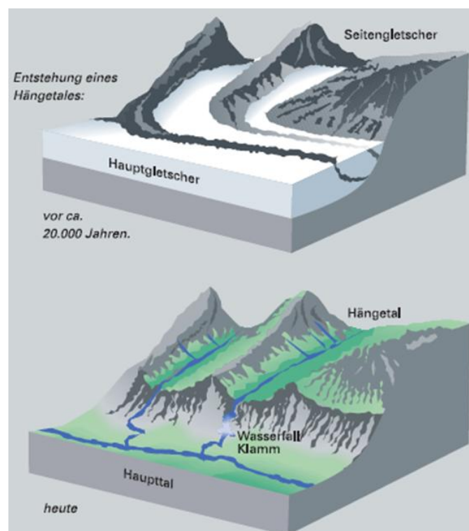
Bild 3: Entstehung eines Hängetales – geologische Erklärung der Klambildung
