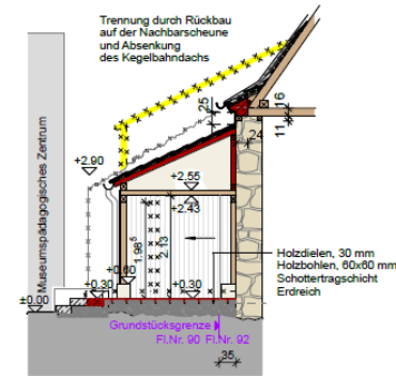
Schnitt A-A
