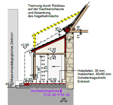
Schnitt A-A
