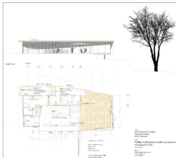
Planzeichnung Gastraum Naturbad Freibergsee
