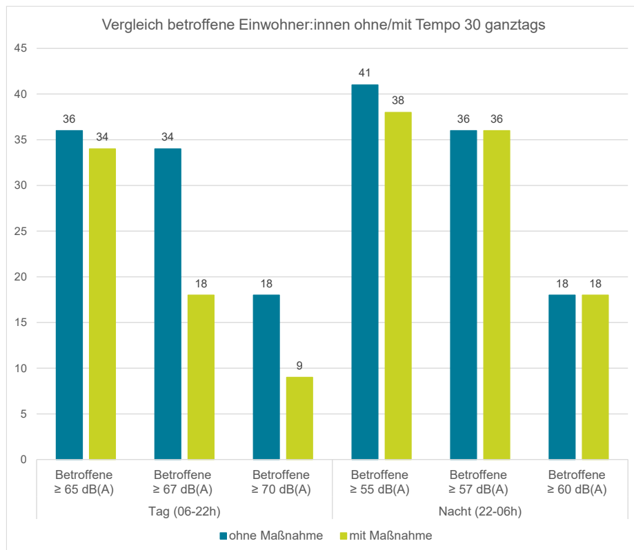
Abbildung 20: Vergleich Lärmbetroffenheiten B 12 Großholzleute, mit/ohne Tempo 30 ganztags
