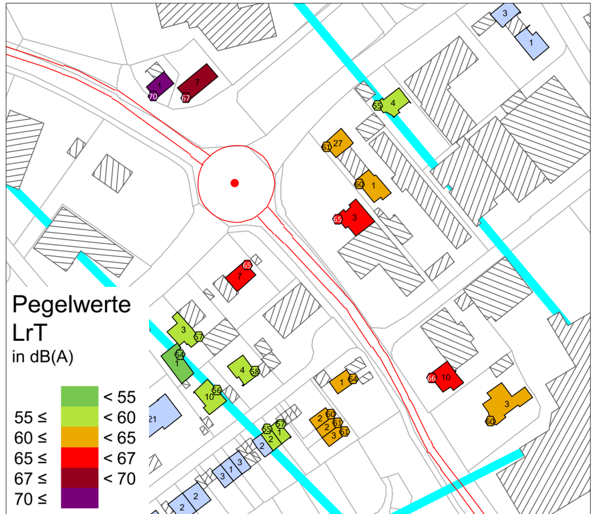
Abbildung 13: Gebäudelärmkarte Tag, L 318 Isny im Allgäu (Ausschnitt)
